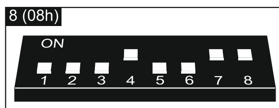
Rys. 10. Sposób ustawienia przełączników DIP-switch w kontrolerze ACU-100.
