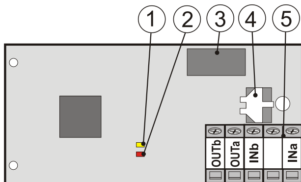
Rysunek: 1 – żółta dioda LED - wskaźnik błędu, 2 – czerwona dioda LED - aktywność; 3 - przełącznik telefoniczny; 4 - elementochrony przeciwprzebiegowej; 5 - zaciski do podłączenia linii telefonicznej uziemienie
