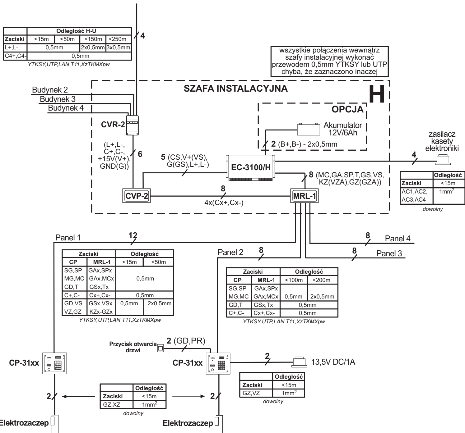
Dobór przewodów dla domofonu CD-3100 w wersji wideo - część 2.
