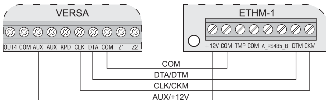
Rys. 12. Sposób podłączenia modułu ETHM-1. Jeżeli centrala ma być zdalnie programowana przez sieć Ethernet, dodatkowo należy przy pomocy produkowanego przez firmę SATEL kabla PIN5/RJ-TTL połączyć port RS-232 modułu ETHM-1 (gniazdo typu PIN-5) z portem RS-232 (TTL) centrali (gniazdo typu RJ).
