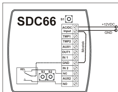
Rys.3 Zasilanie SDC66 z sieci prądu stałego DC
