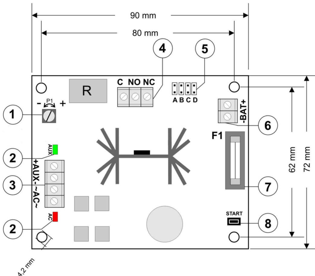
Rys.2. Widok modułu zasilacza.
