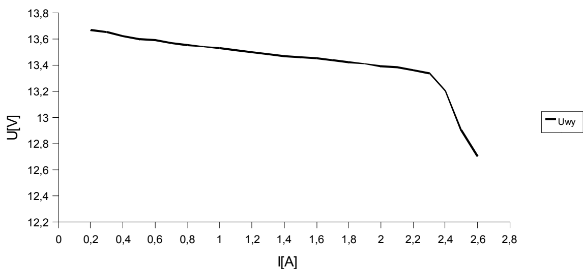
Rys. 2. Charakterystyka prądowo-napięciowa zasilacza.
