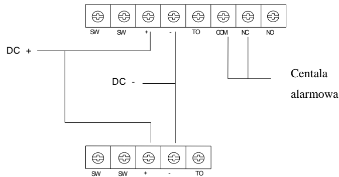
Przykładowe podłączenie
